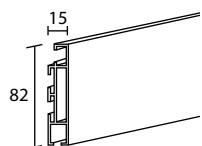
853300 Profilo frontale Frontal profile Profil frontal Blende Perfil frontal Profil przedni
