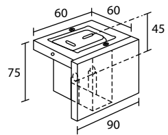
863414 Intermedio P/P Middle P/P Intermédiaire P/P Mittelträger P/P Intermedio P/P Środkowy P/P
