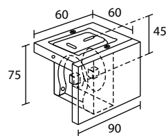
863425 Intermedio C/C Middle C/C Intermédiaire C/C Mittelträger C/C Intermedio C/C Środkowy C/C
